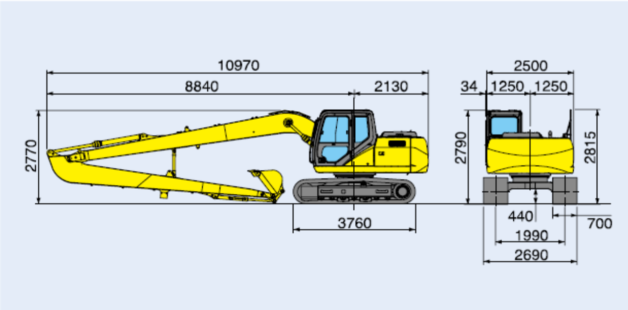
外形寸法図
