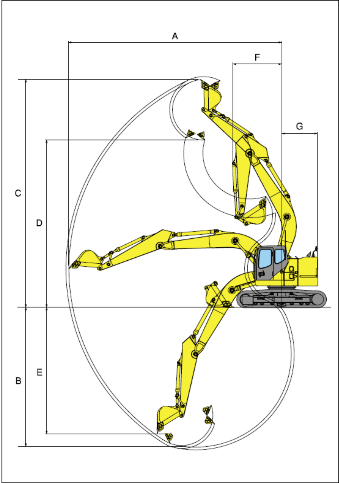
作業範囲図
