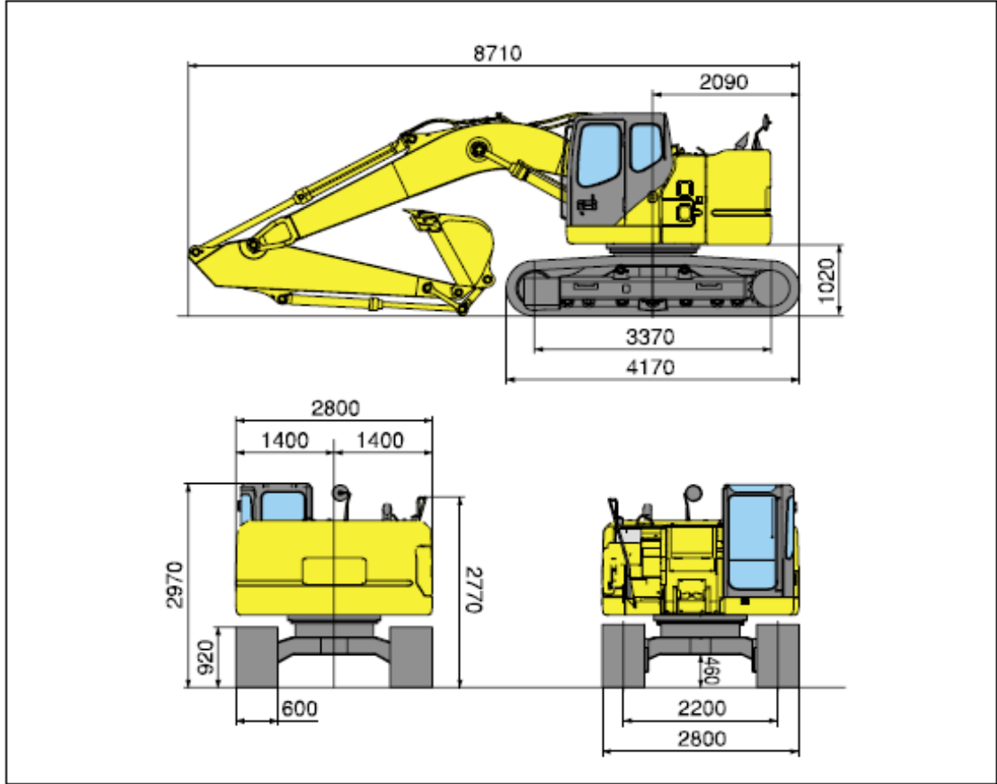
外形寸法図
